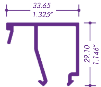
1105 / 71256 JUNQUILLO 14 MM
