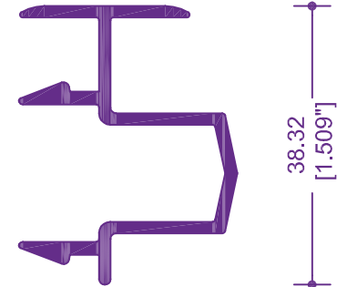
1543 / 64206 ADAPTADOR OXXO
