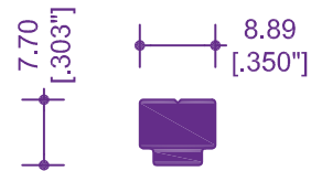
8035 / 14412 CONECTOR
