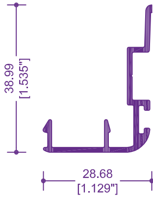
8018 / 62002 TRASLAPE
