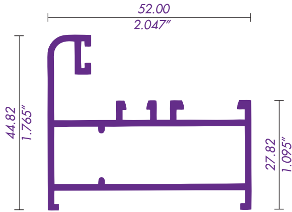
4525 / 62033 "L" CONTRAMARCO
