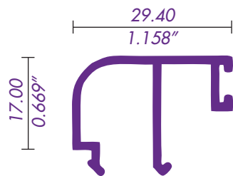
4594 / 62029 JUNQUILLO 6mm.
