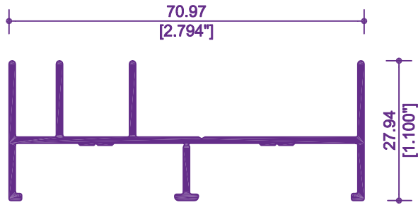
7040 /78408 JAMBA
