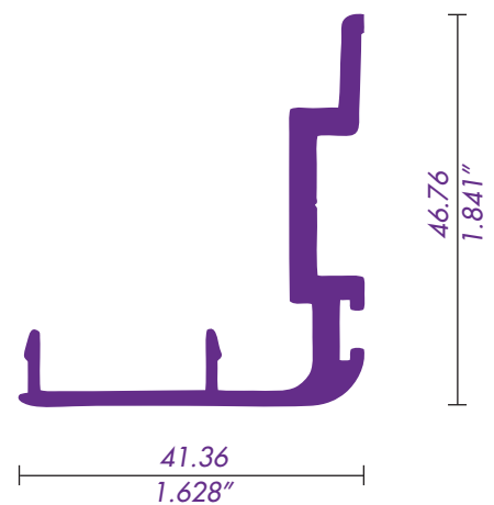
1518 / 62058 TRASLAPE
