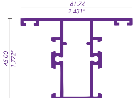
4521 / 62041 INTERMEDIO CUADRÍCULA
