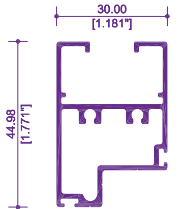
3504 / 12276 MARCO
