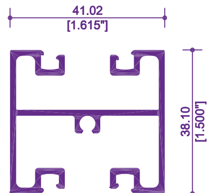
1021 / 14409 INTERMEDIO
