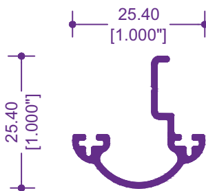
5084 / 12653 ADAPTADOR INTERMEDIO
