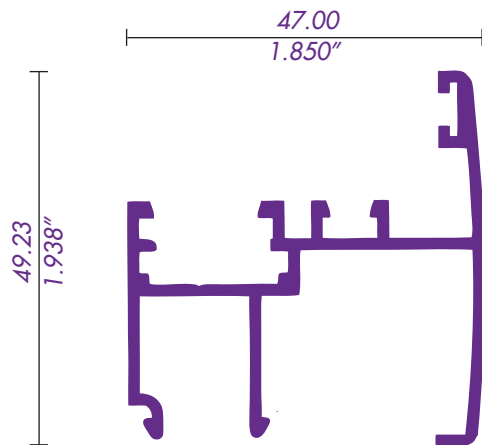
4528 / 62031 INTERMEDIO MÓVIL
