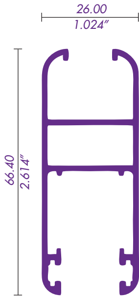
8017 / 62001 CERCOS 6mm
