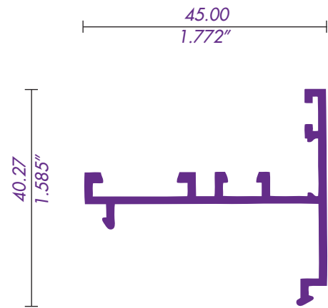
4522 / 62032 CONVERTIDOR
