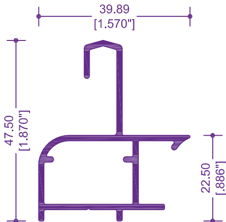
8021 / 64207 ADAPTADOR RIEL
