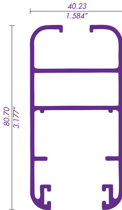
1517 / 62055 CERCO 6mm
