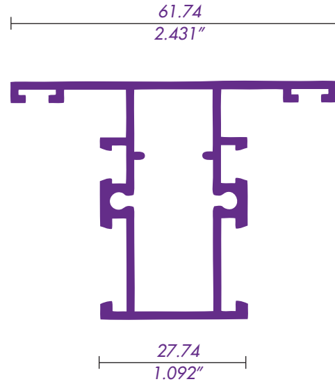
4521 / 62041 INTERMEDIO CUADRICULA
