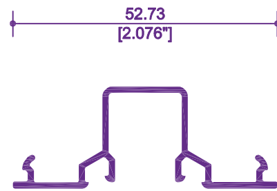
5027 / 12505 TAPA BOLSA
