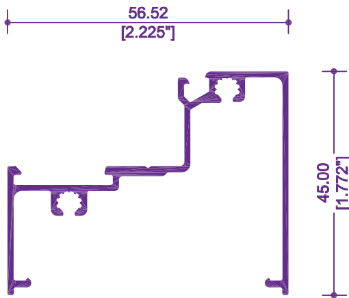
5022 / 12506 ESCALONADO EXTERIOR
