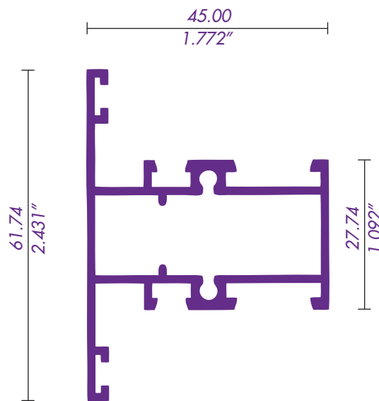
4521 / 62041 INTERMEDIO CUADRICULA
