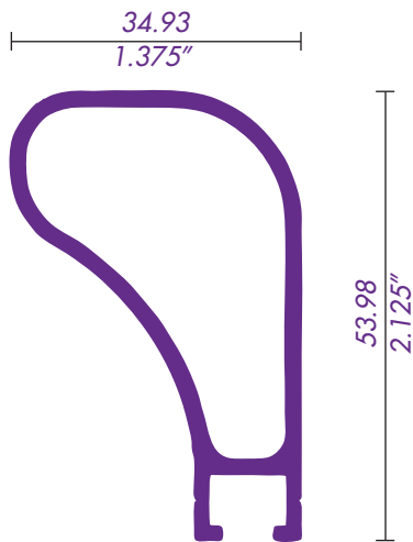
8034 / 62014 REFUERZO
