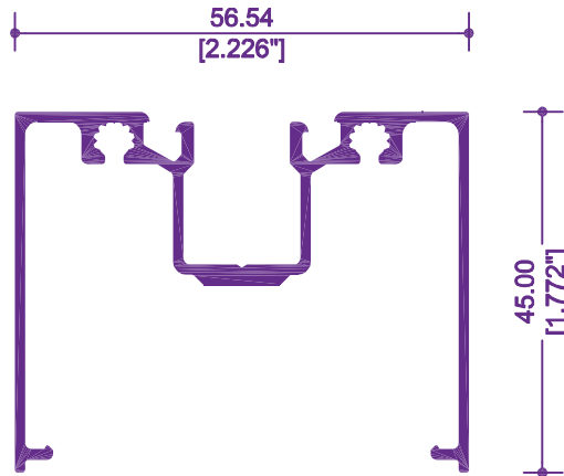
5025 / 12504 BOLSA
