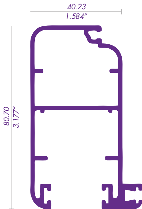
1512 / 62057 MOSQUITERO
