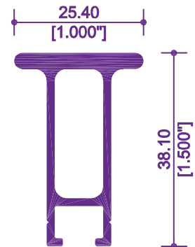
7038 / 14411 REFUERZO 1 1/2"
