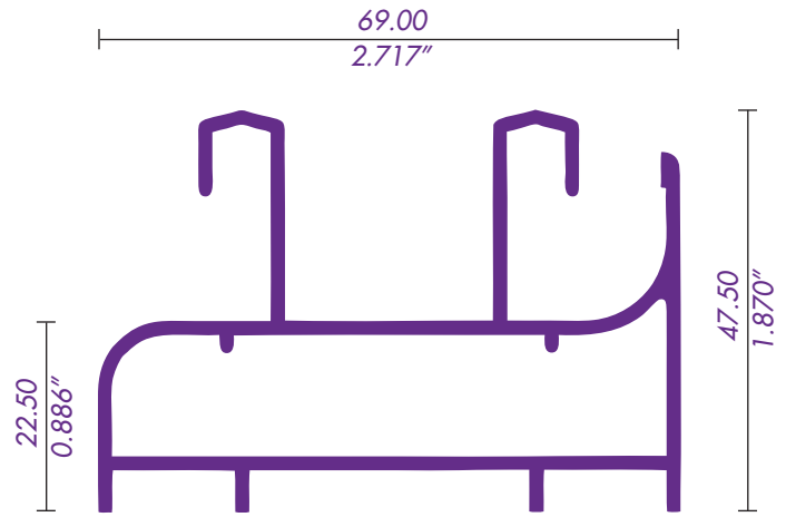
8019 / 62000 RIEL BASICO
