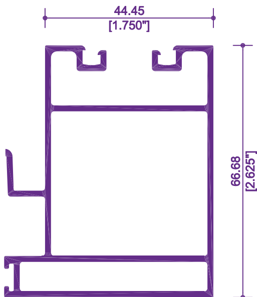
1018 / 14427 CERCO TRASLAPE
