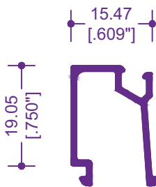
5093 / 12543 JUNQUILLO
