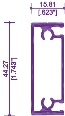
7084 / 11411 MOSQUITERO
