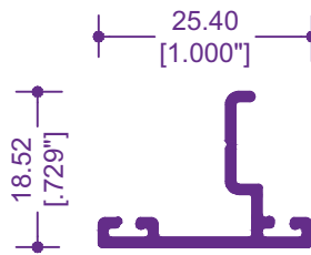
5082 / 74272 TOPE RECTO
