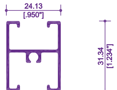
7045 / 12456 INTERMEDIO
