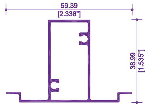
3502 / 12275 INTERMEDIO
