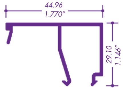
1104 / 71255 JUNQUILLO 6 MM
