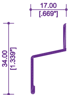
7081 / 12428 BOTAGUAS
