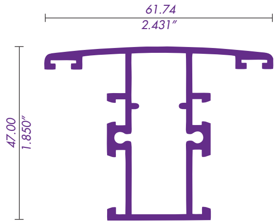
4524 / 62028 "T" INTERMEDIO
