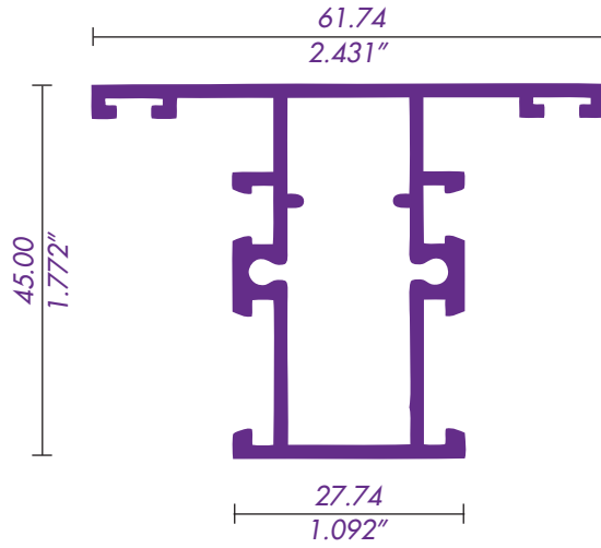
4521 / 62041 INTERMEDIO CUADRÍCULA
