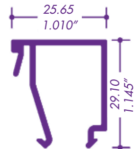
1106 / 69920 JUNQUILLO 24 MM
