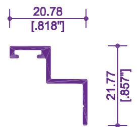
5043 / 50701 ADAPTADOR OXXO
