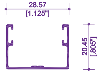
7082 / 18413 GUÍA INFERIOR
