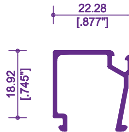
5023 / 12507 JUNQUILLO
