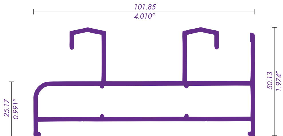
1519 / 62052 RIEL DOBLE
