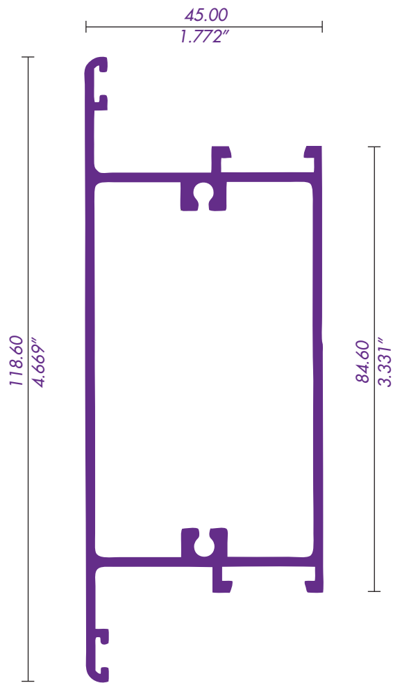
4592 / 62039 INTERMEDIO
