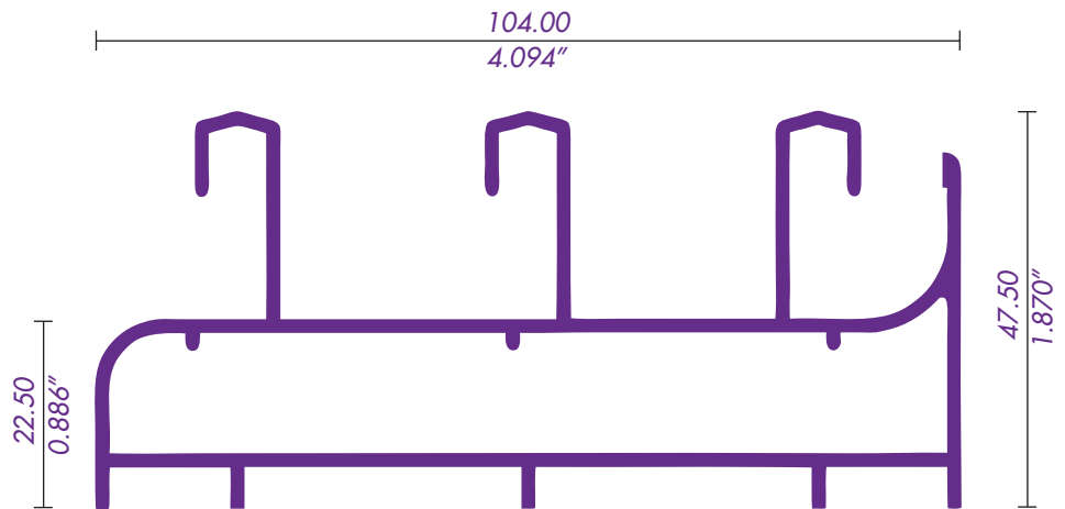
8029 / 62017 RIEL TRIPLE
